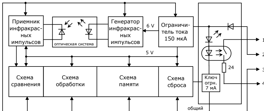
Рисунок 1 - Структурная схема ИП212-54Р
