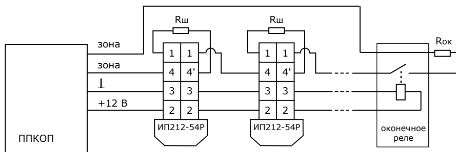
Рисунок 7 - Схема подключение извещателей ИП212-54Р1 к ППКОП с использованием оконечного реле для контроля наличия напряжения питания
